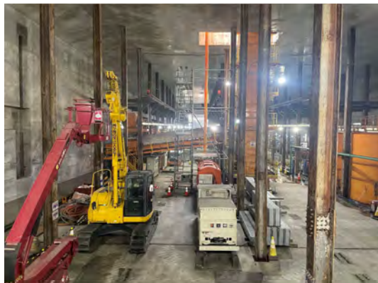
シールドマシン後方設備の状況 (令和7年7月7日)
