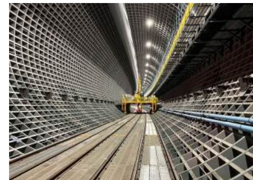
構築されたトンネル内(鋼製セグメント) (令和7年7月25日)
