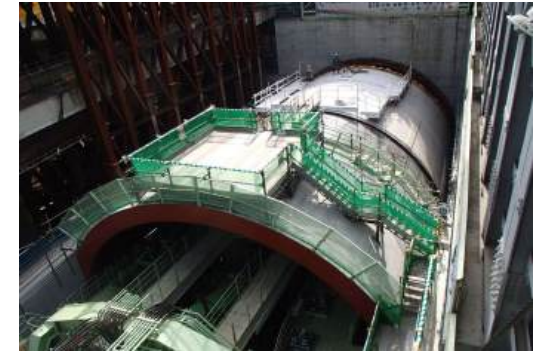
シールドマシン組立完了状況 (平成31年1月27日)
