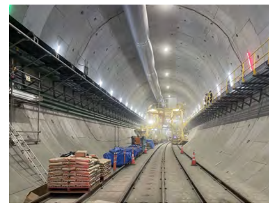
シールドトンネル坑内の状況 (令和7年11月24日)
