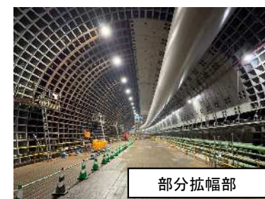
東名JCT地中拡幅(南行)の現地状況
