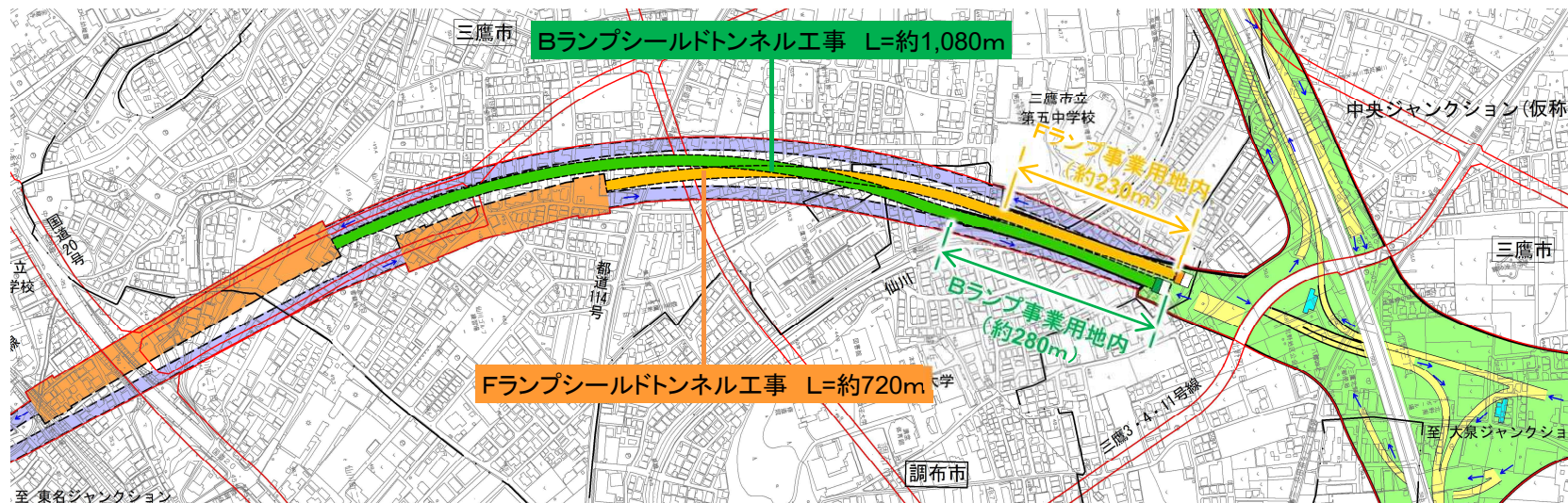
東名JCT Hランプの掘進実績(事業用地内:134m)約8ヶ月
