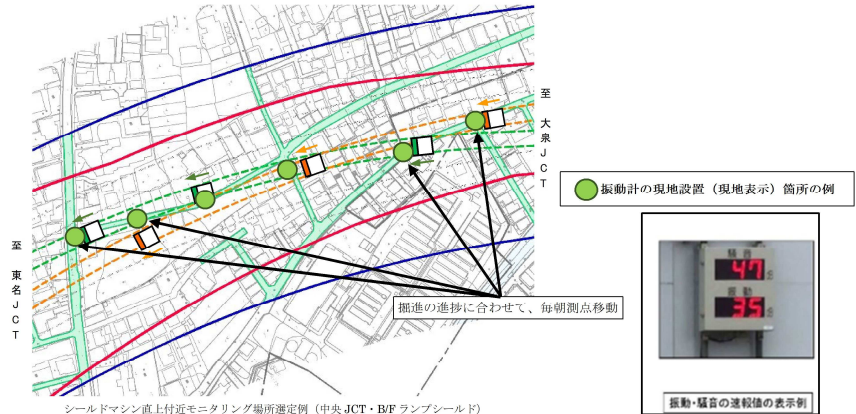
シールドマシン直上付近モニタリング場所選定イメージ
