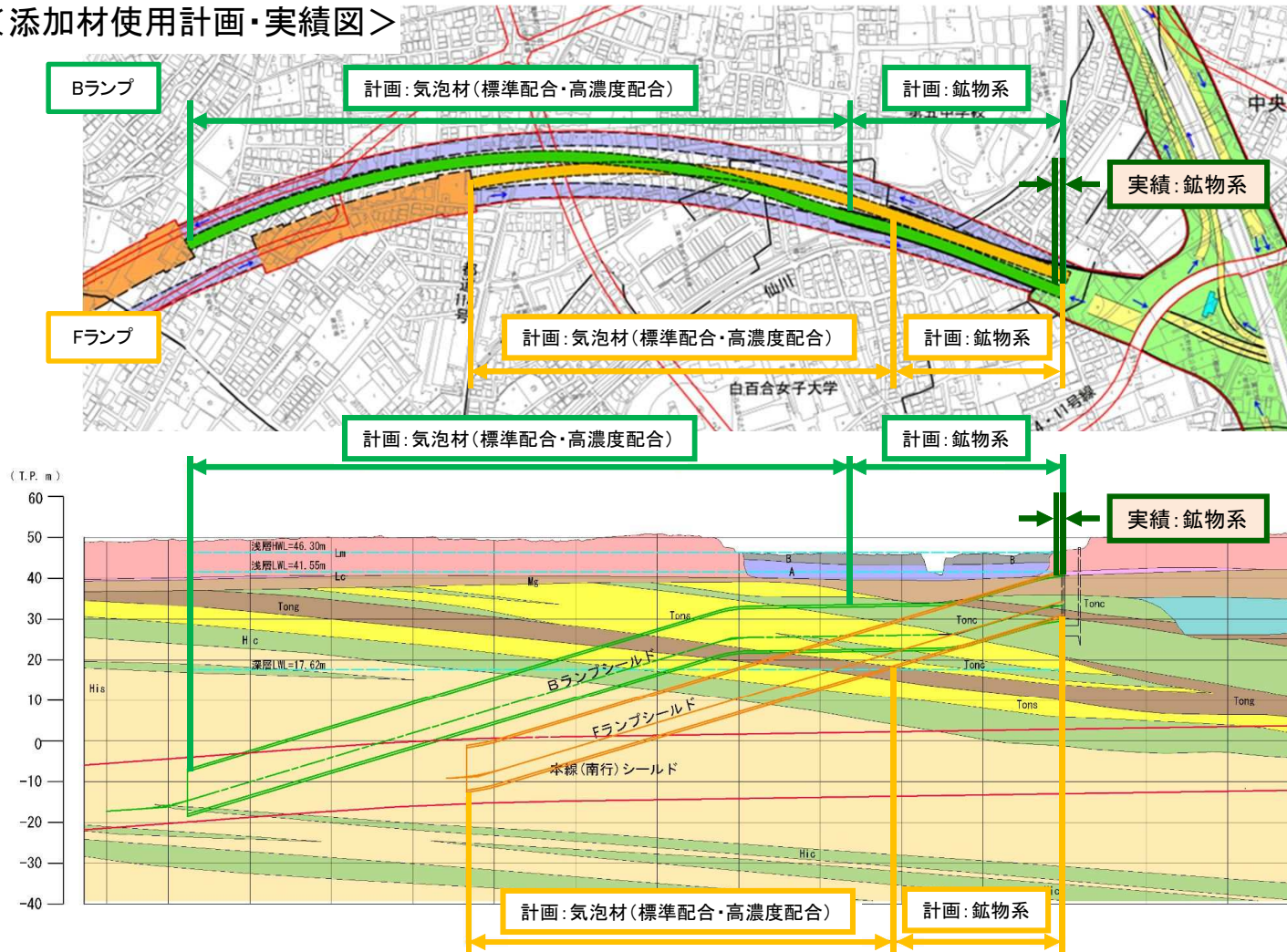
※路線地質縦断面図（平成26年度時点）
