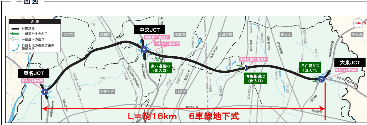
平面図
