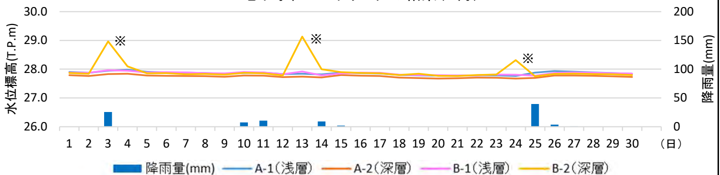
地下水位モニタリングの結果(6月)
