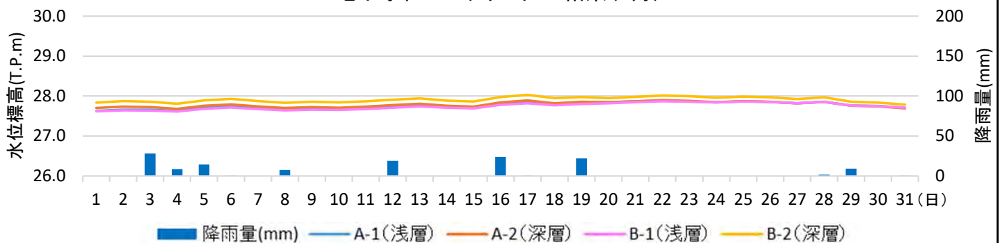
地下水位モニタリングの結果(3月)
