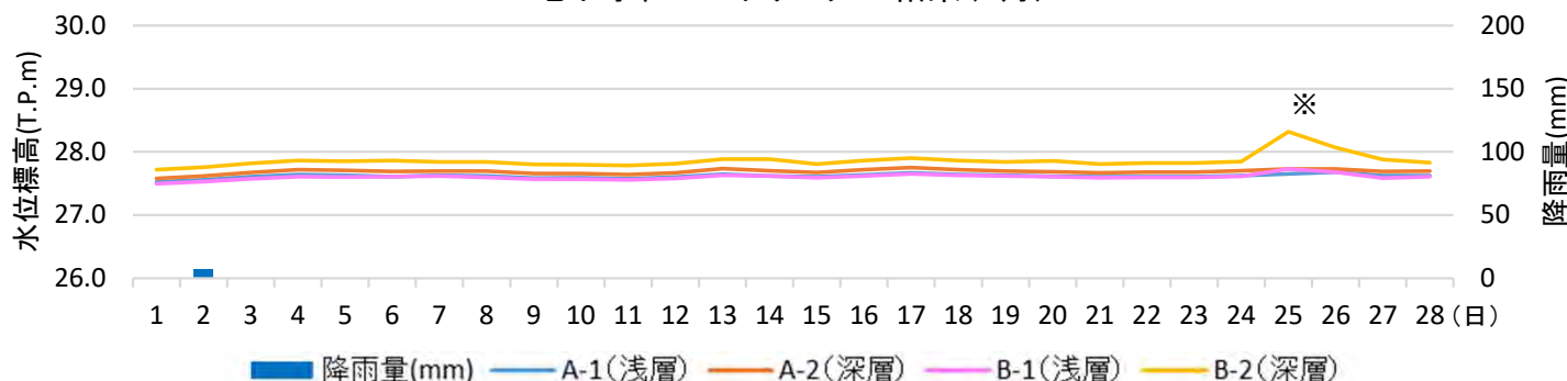
地下水位モニタリングの結果(2月)
