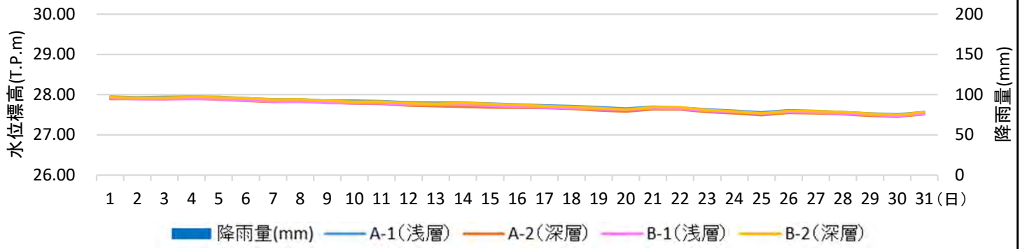
地下水位モニタリングの結果(12月)
