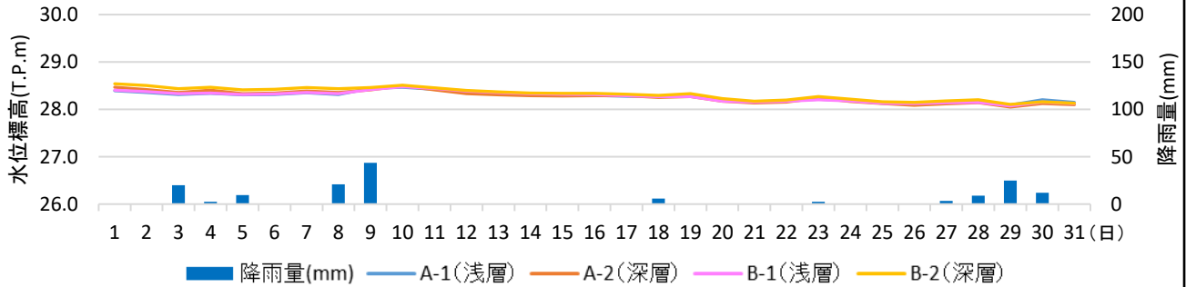
地下水位モニタリングの結果(10月)
