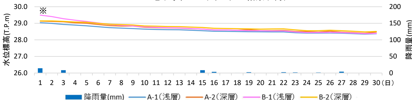
地下水位モニタリングの結果(9月)
