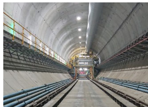
Aランプ坑内(シールド先端部)
