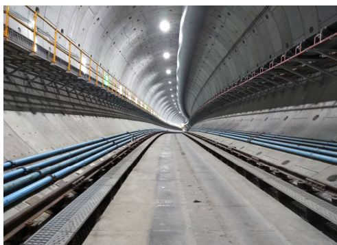
Aランプ坑内(シールド構築状況)
