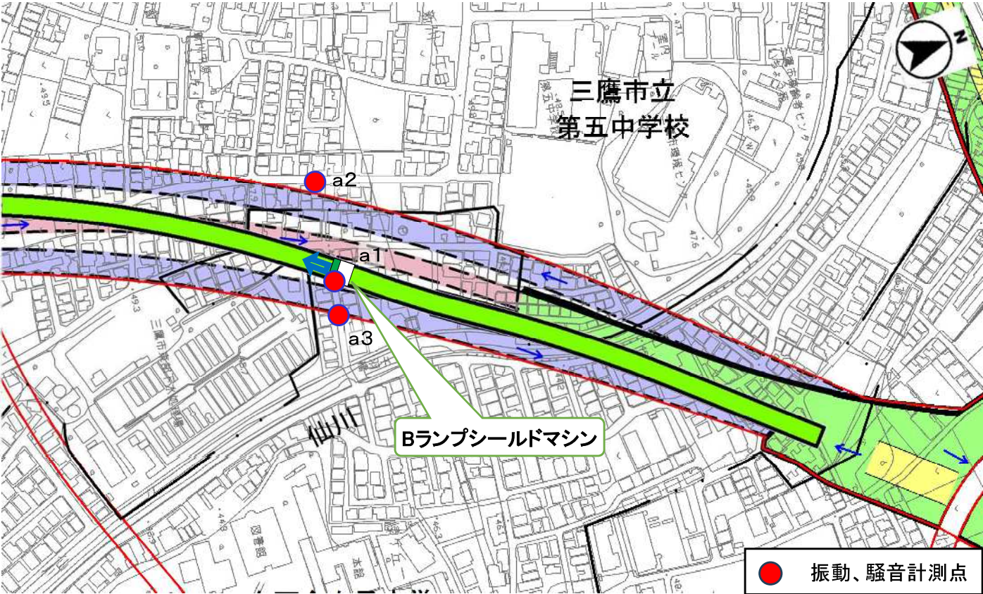
【 10月17日(水)7:30～17:00 振動・騒音計測結果(確定値)】
