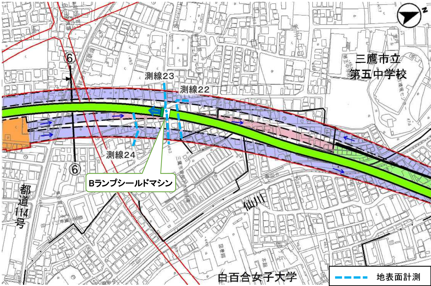
【12月16日(火) 地表面変位計測結果】
