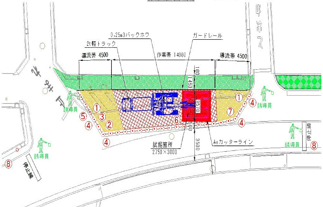
作業帯平面図 S=1:200
